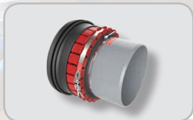
Adaptateur BSM Raccordement sur tulipe béton ou grès DN 250 à 400
